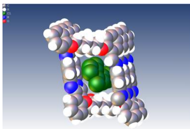
Slika 1. Molekulska struktura spoja s ugrađenim molekulama klora.
