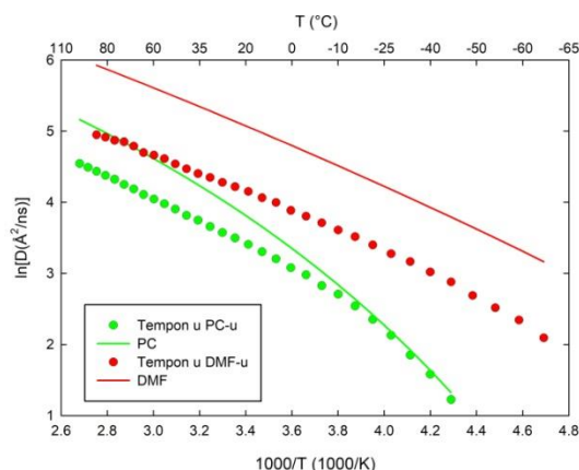
Slika 1. Krivulje difuzivnosti tempona i koeficijenata samodifuzije za PC i DMF
