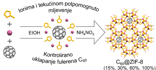
Slika 1. Shematski prikaz sintetskog postupka uklanjanja fulerena C_{60} u ZIF-8
