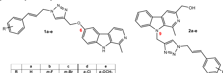
Slika 1. Nova generacija harmicina triazolskog tipa.
