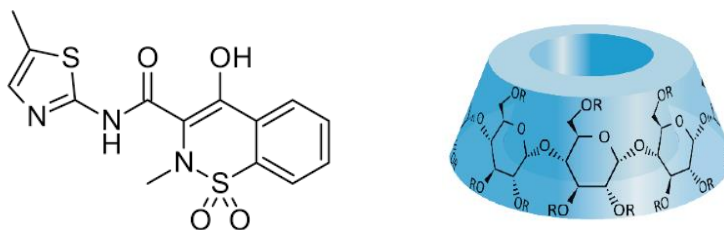
Slika 1. Melosikam i \beta -ciklodekstrin
