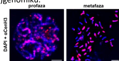
Slika 1. Organizacija centromere u vrsti Meloidogyne incognita . Imunofluorescencija \alpha CenH3-pripadajućih domena (crveno) s kromosomima koji su obojani DAPI bojom (plavo), mjera=5 \mu m.
