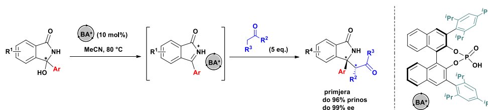
Slika 1. Stereoselektivna priprava \beta,\beta -diaril-ketona s \beta -kvaternim stereogenim centrom katalizirana kiralnom Brønstedovom kiselinom.
