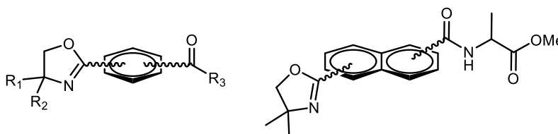
Slika 1. Ligandi s benzenskom (lijevo) i naftalenskom (desno) centralnom strukturnom jedinicom različitih supstitucijskih motiva (lijevo: 1,3-, 1,4-; desno: 1,4-, 1,5-, 2,6-, 2,7-). R 1 = Me, i-Pr, Ph, Bn, R 2 = H, Me, R 3 = NH-Ala-OMe, NH-Gly-Val-Phe-OMe.
